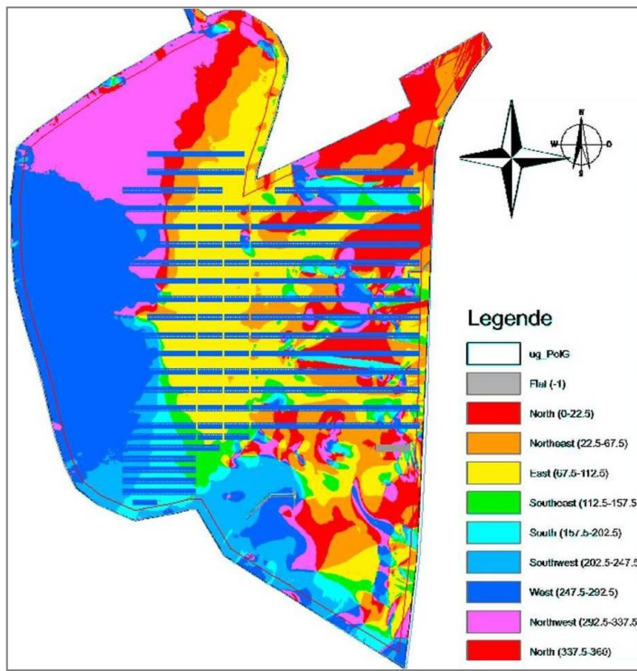
Bild 5: Geländeausrichtung
