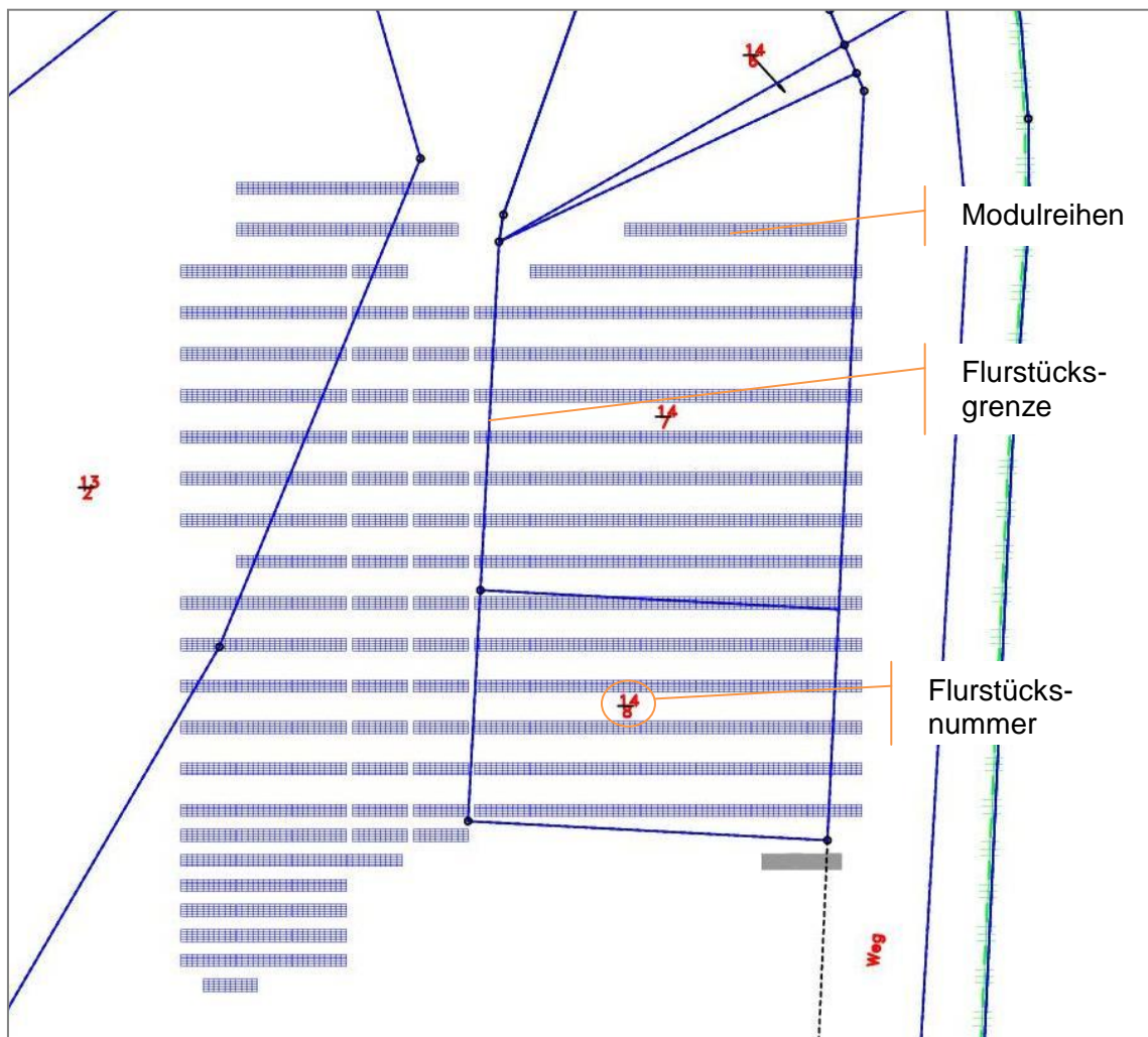
Bild 4: Flächenbelegung, schematisch
